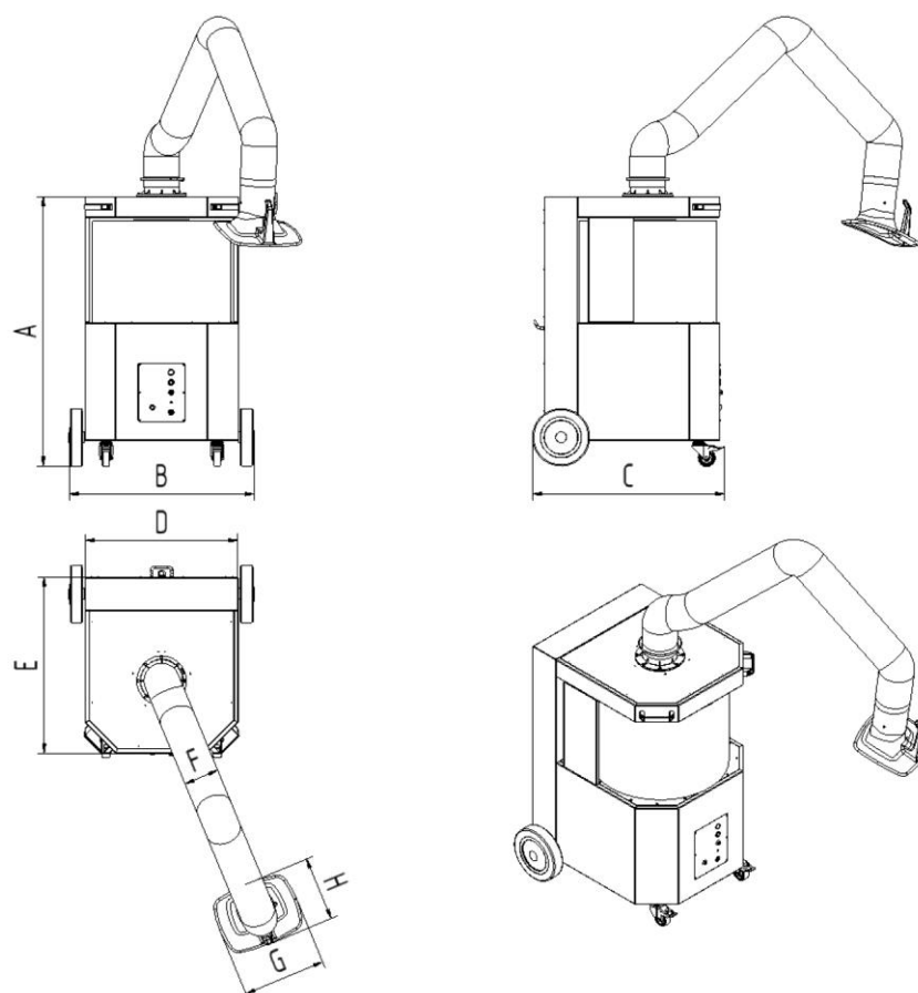
Rys. 7: Karta wymiarów
